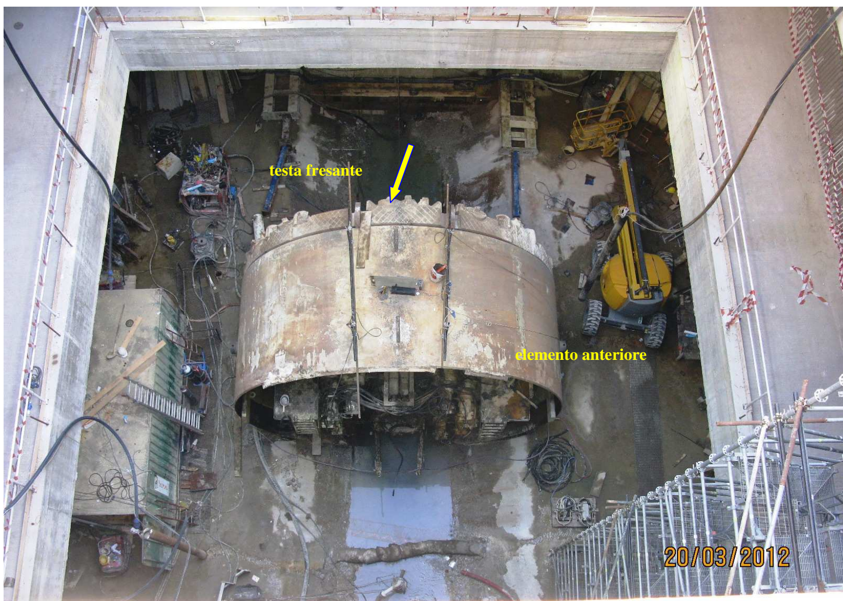
Pozzo di estrazione della TBM a Municipio
