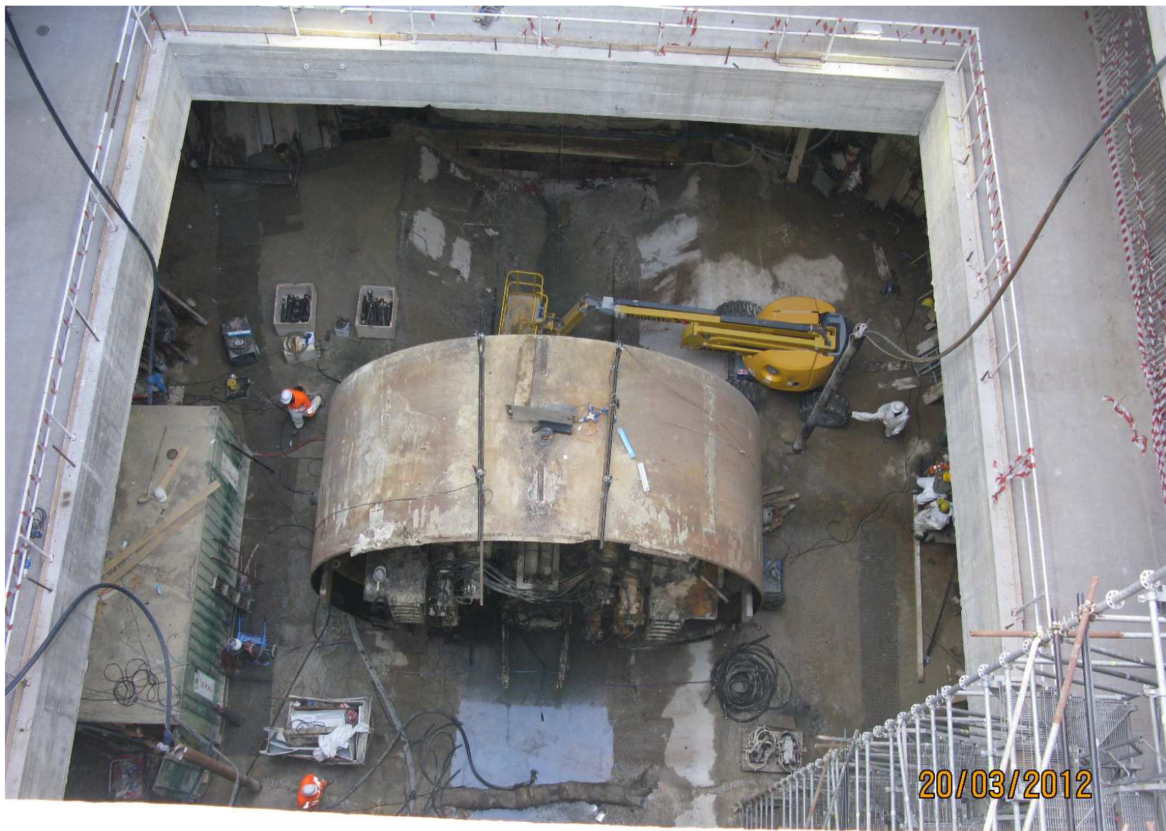
Pozzo di estrazione della TBM a Municipio Elemento anteriore da estrarre ( peso c.a. 260 tonn. )
