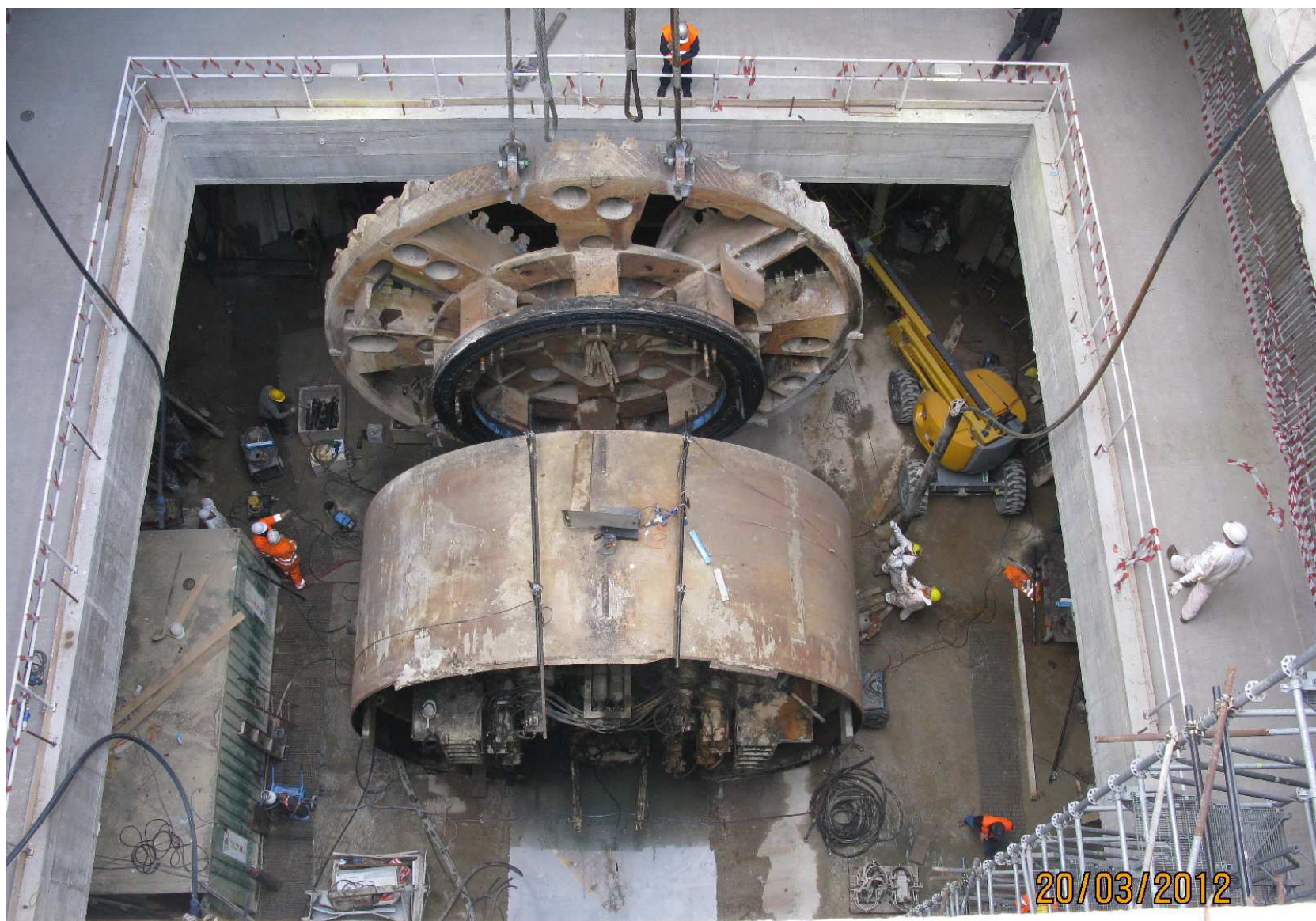
Pozzo di estrazione della TBM a Municipio Ultimato lo scollegamento della testa fresante dall'elemento intermedio
